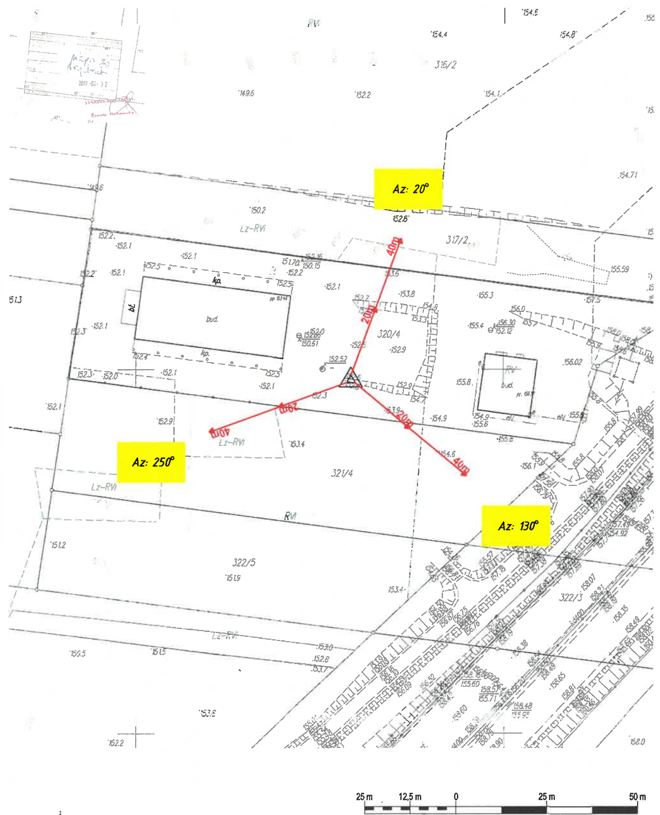
Rys. 1. Rzut poziomy osi głównej wiązki promieniowania w odległości do 20 i 40 metrów od środka elektrycznego anten.
